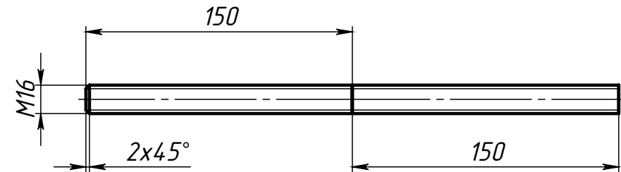
Поз.4 и Поз.8 (Шпильки резьбовые) 1 : 3
