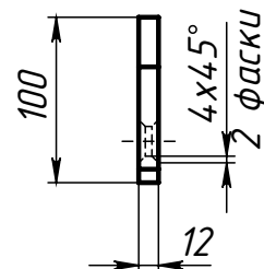
Поз.9 (Серьга) 1 : 5
