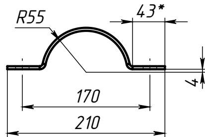
Поз.10 (Полухомут) 1 : 5
