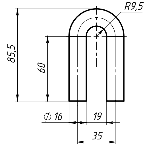
Поз.2 (Ушко) R9,5
